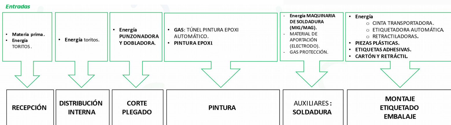
Ejemplo Diagrama de flujos de una empresa analizada en el 4º proyecto de EC
